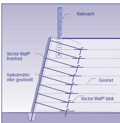
Vector Wall® som grøn støttemur med traditionelt rækværk.
